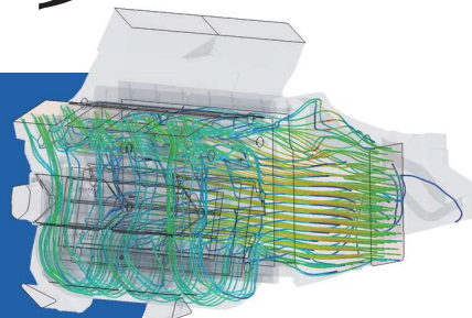
ヒーターユニット内部の風の流れ解析
